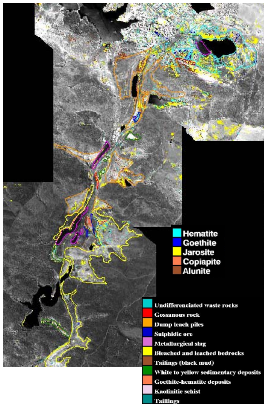
Figura 8. Detecção de minerais geradores de Drenagem Ácida Mineira. Resultados obtidos pela intersecção dos algoritmos SAM e MTMF utilizando bibliotecas standardizadas (USGS). Linhas correspondem a cartografia de campo (legenda inferior).
