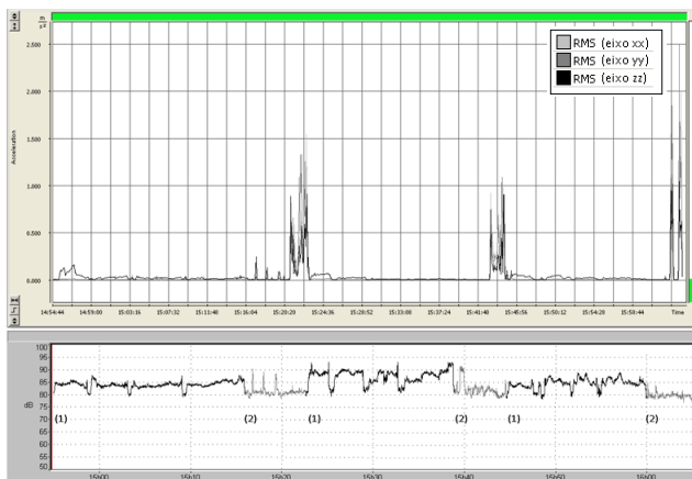
Figura 1 - Vibrações vs. Ruído carro perfuração
