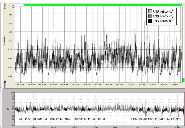
Figura 2 – Vibrações vs. Ruído giratória c/ balde
