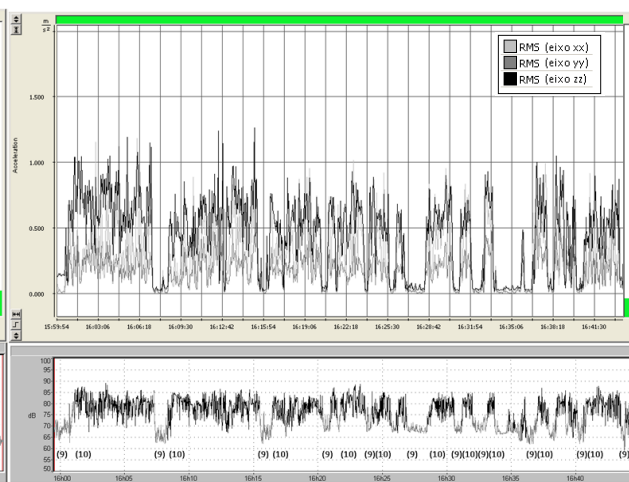
Figura 4 - Vibrações vs. Ruído giratória c/ martelo hidráulico.
