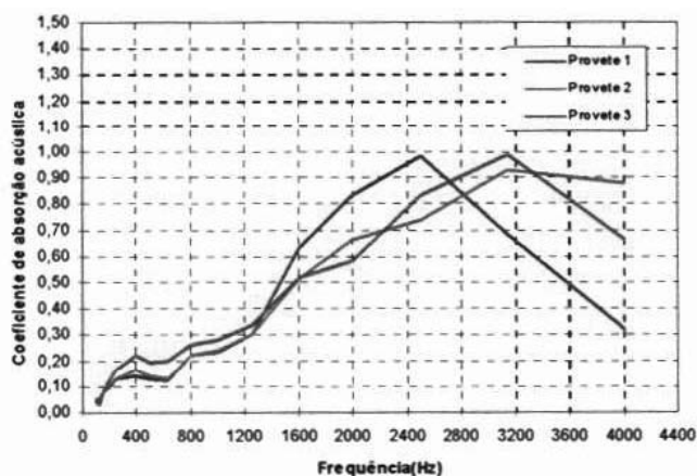
Gráfico 1. Absorção acústica em função da frequência.
