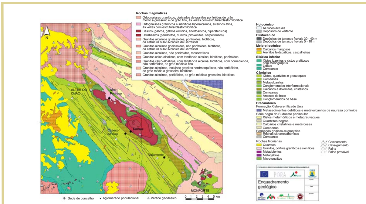
FIGURA 3 - Enquadramento geológico da região de Monforte-Alter do Chão
