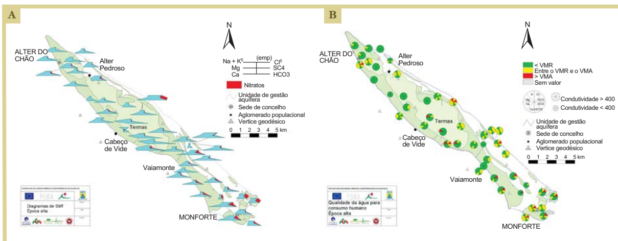
FIGURA 7 - Época de águas altas de 1997/1998: A - Diagramas de Stiff e B - Qualidade da água para consumo humano segundo os valores máximos recomendáveis (VMR) e admissíveis (VMA) definidos no Decreto-Lei nº 236/98, de 1 de Agosto
