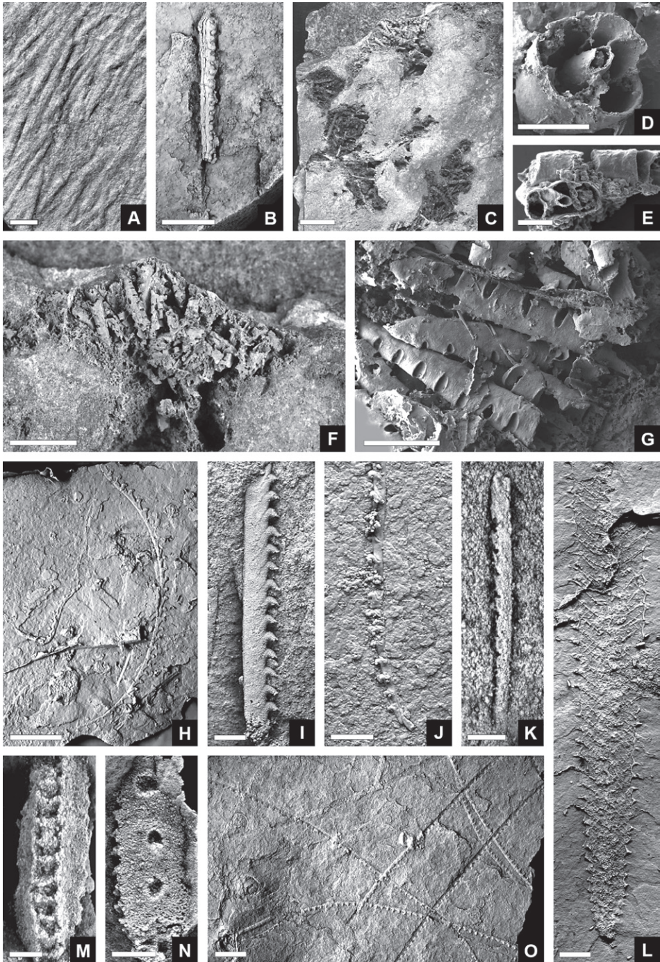
Fig. 2. Graptolitos silúricos procedentes de varios yacimientos ubicados en los sinclinales de Almadén (A, C-G), Guadalmez (H, L), Herrera del Duque (I, K, M-N), Corral de Calatrava (J, O) y Sierra Morena Oriental (B). A-G, graptolitos aeronienses procedentes de la parte alta de la Cuarcita de Criadero; H-L, formas del Telychiense o
