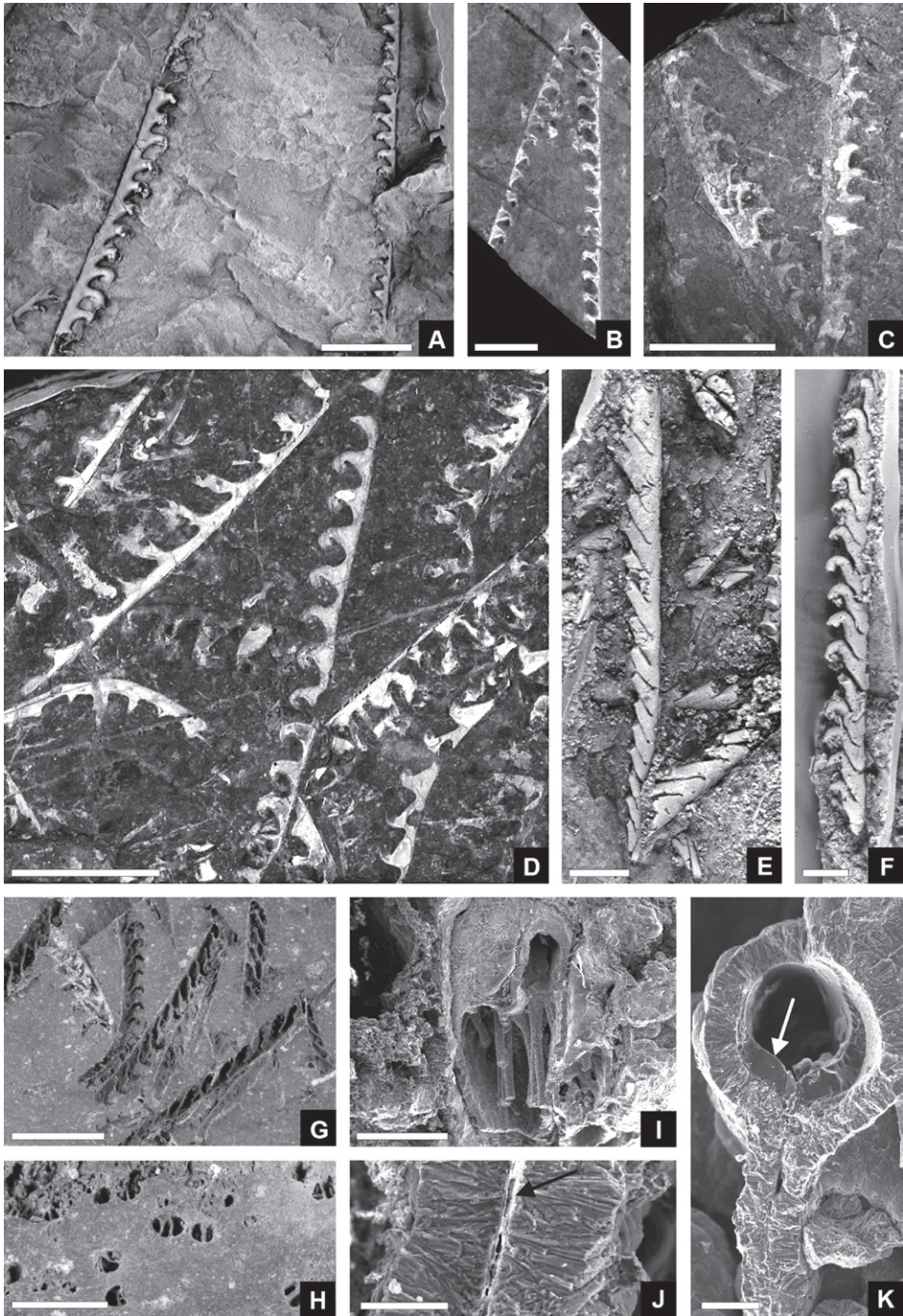
Fig. 1. Graptolitos del Silúrico portugués conservados en liditas del Aeroniense del anticlinal de Valongo (A-D: PIÇARRA et al. , 2009) y en nódulos silico-fosfatados del Sheinwoodiense del sinclinal de Moncorvo (E-K: SÁ et al. , 2009). A. Vaciado en látex de dos fragmentos de rabdósomas. B, D. monograptidos con recristalización
