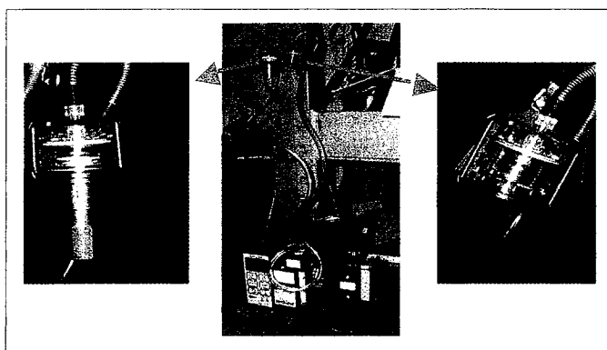
Figura 1 – Exemplo de montagem com 2 bombas de amostragem para recolha da fracção respirável em ciclone de alumínio (detalhe à esquerda) e fracção inalável em cassette (detalhe à direita).
